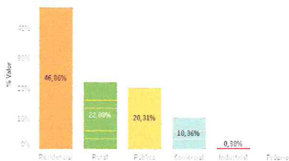
Gráfico 3.3.1 – Consumo de energia elétrica, por classes de consumo (mwh) - 2019
